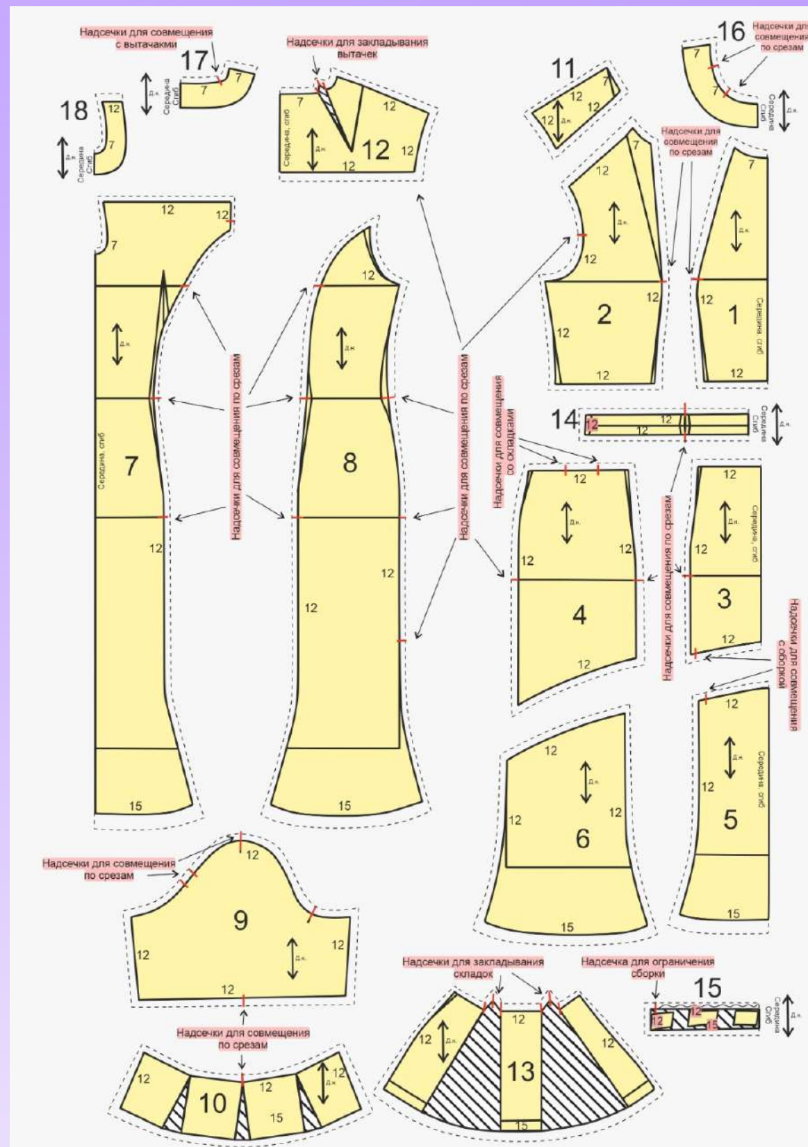
Конструктивное моделирование
